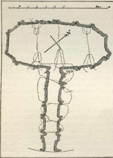
Grundplan af Møllehøj. (Efter Arkitekt E. Schiødtes Opmaaling.)
